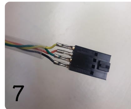
connecteur C-GRID vu de face
