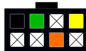
connecteur C-GRID vu de face
