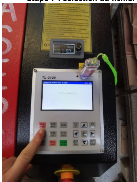
Mettre la clé USB dans la machine et appuyer sur le bouton "Reset". La machine se remet à zéro.
