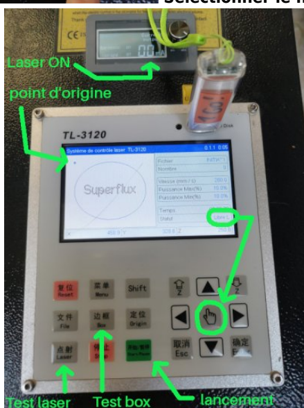
Sélectionner le fichier en appuyant sur le bouton "enter".
